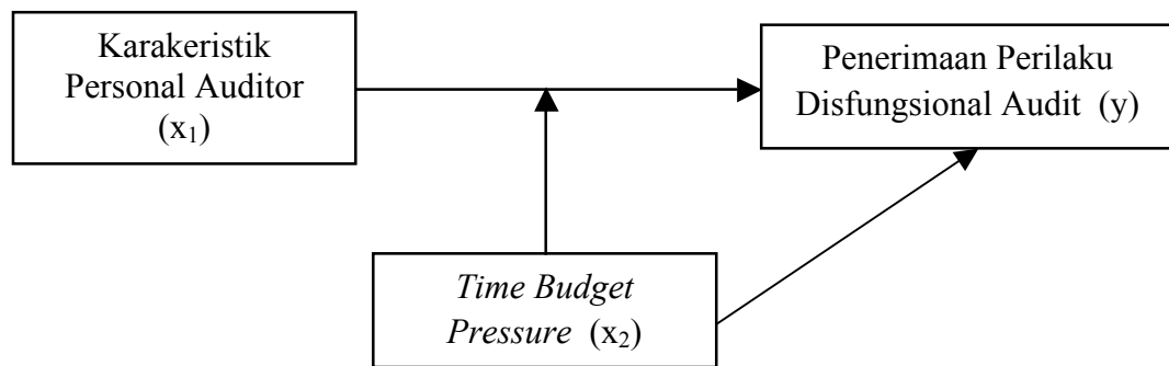
Gambar 1. Kerangka Konseptual
