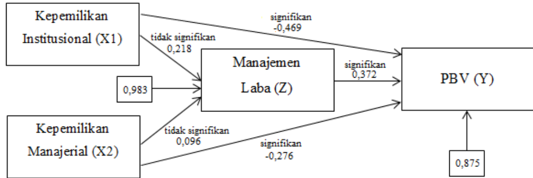
Gambar 1. Diagram Hasil Analisis Jalur
