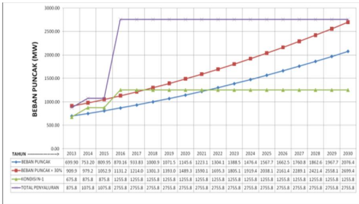
Gambar 4. Grafik Neraca Daya Sistem Kelistrikan Bali Skenario 1
