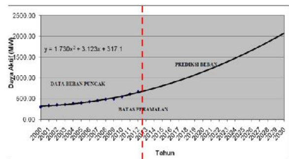
Gambar 3. Prediksi Beban Puncak Sistem Kelistrikan Bali tahun 2000-2012
