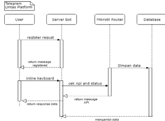
Gambar 3 Sequence Akses Data API Mikrotik dan database
