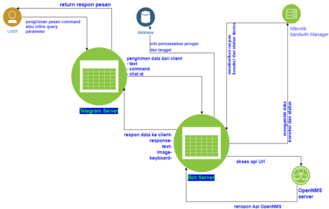
Gambar 1 Arsitektur Sistem
