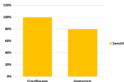
Gambar 4. Sensitivitas Enterococcus faecalis terhadap beberapa antibiotik
