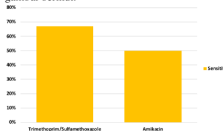
Gambar 3. Sensitivitas Acinetobacter baumannii terhadap beberapa antibiotik
