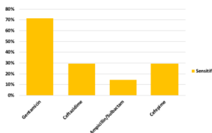
Gambar 2. Sensitivitas Klebsiella pneumoniae terhadap beberapa antibiotik
