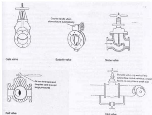
Gambar 1: Jenis-jenis katup[9]
