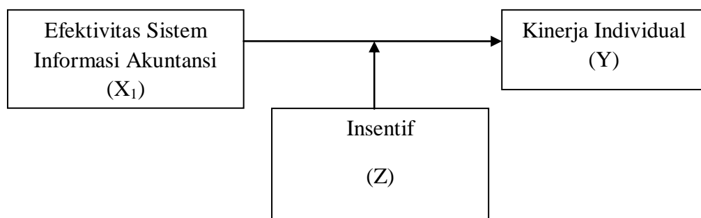
Gambar 1. Desain Penelitian
