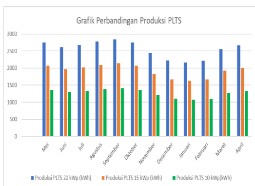
Gambar 7. Perbandingan produksi PLTS dari 3 Skenario
