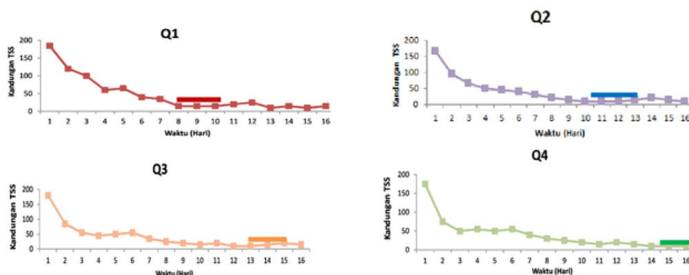
Gambar 2. Penurunan TSS selama proses aklimatisasi, dimana Q1 : Laju Aliran limbah 50 ml/menit, Q2 : Laju Aliran limbah 100 ml/menit, Q3 : Laju Aliran Air Limbah 150 ml/menit, dan Q4 : Laju Aliran Air Limbah 200 ml/menit.
