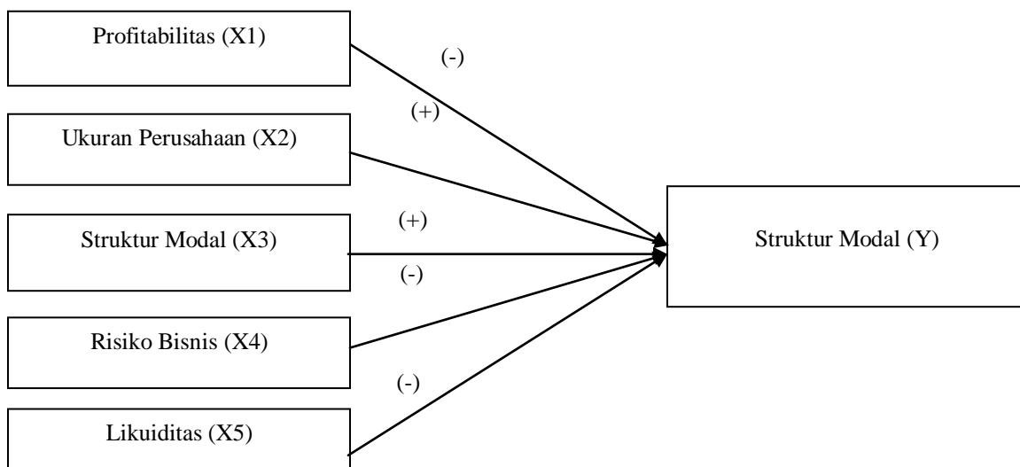
Gambar 1. Desain Penelitian
