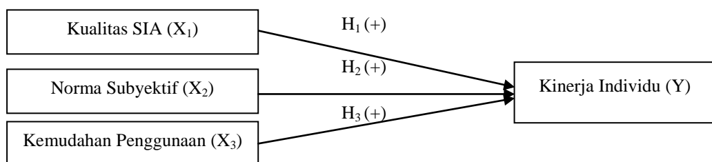
Gambar 1. Desain Penelitian
