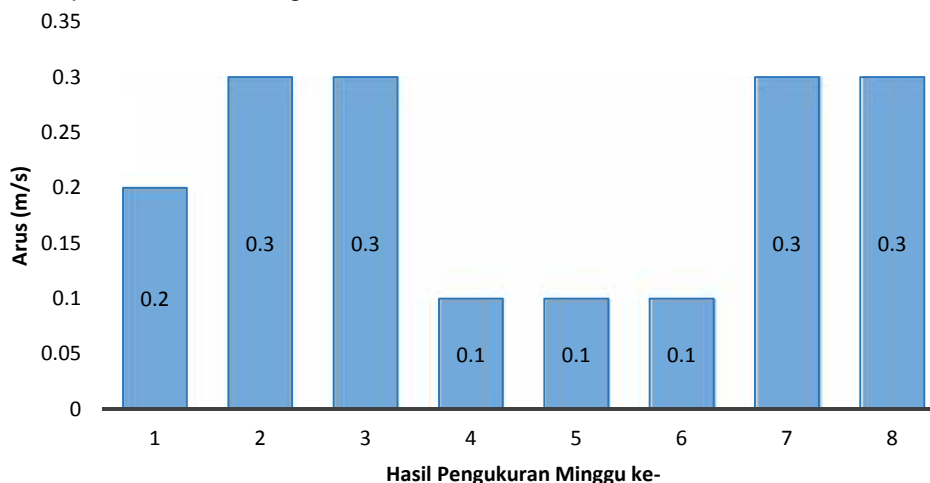
Gambar 5. Hasil Pengukuran Arus di Perairan Kutuh
