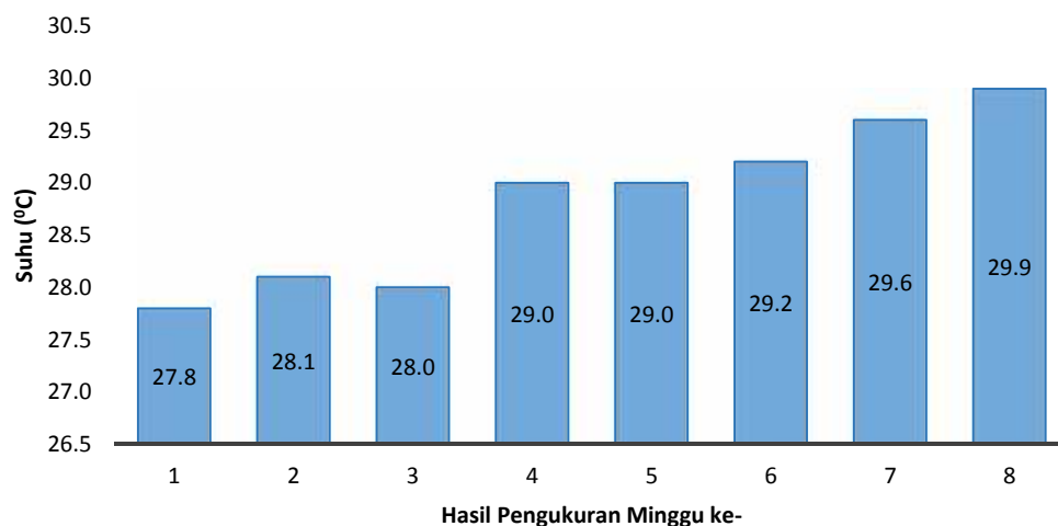
Gambar 1. Hasil Pengukuran Suhu di Perairan Kutuh
