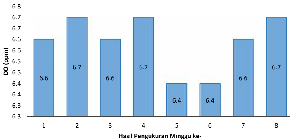
Gambar 2. Hasil Pengukuran DO di Perairan Kutuh
