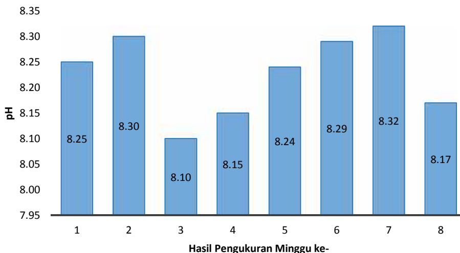
Gambar 4. Hasil Pengukuran pH di Perairan Kutuh
