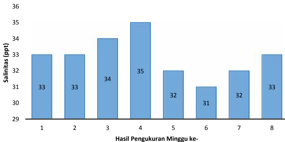
Gambar 3. Hasil Pengukuran Salinitas di Perairan Kutuh
