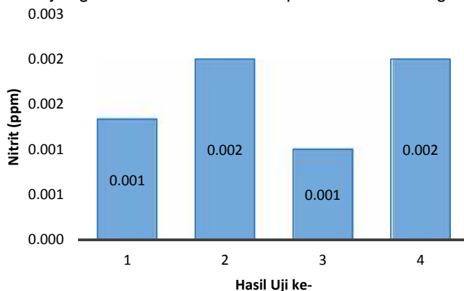
Gambar 7. Hasil Pengukuran Nitrit
